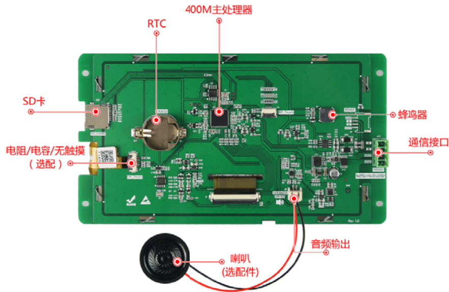
图 1-4 硬件配置图
